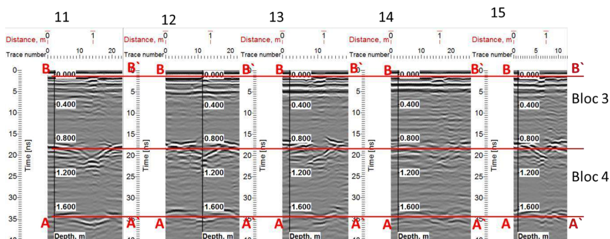
Figura 9 Radargrame efectuate pe lățimea coloanei 1, față "b"
