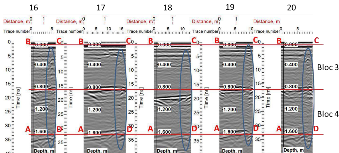
Figura 8 Radargrame efectuate pe înălțimea coloanei 1, față "b"
