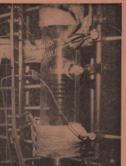
Conversia MHD în condiții de conversie continuă. Se observă sistemul de alimentare cu gaze și sistemul de răcire.
